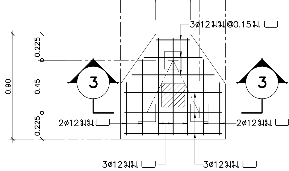
แปลนแสดงการเสริมเหล็ก มาตราส่วน 1 : 20
