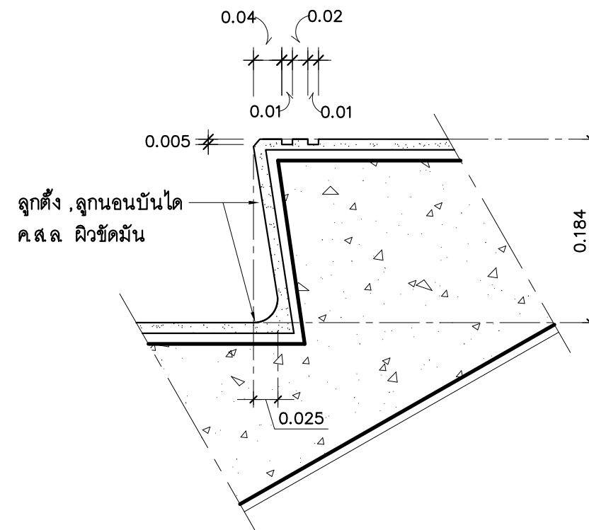
แบบขยายจมูกบันได
