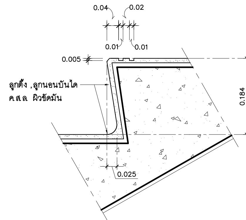
แบบขยายจุ่มบันได มาตราส่วน 1 : 5
