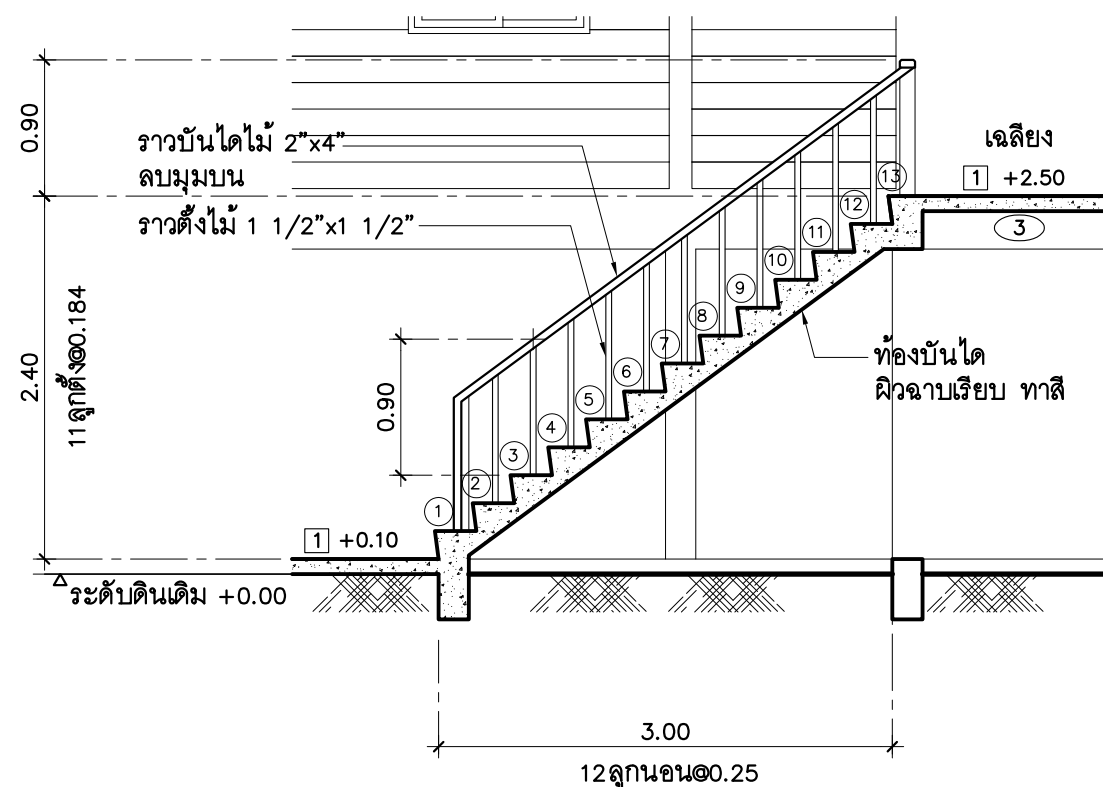
รูปตัด มาตราส่วน
