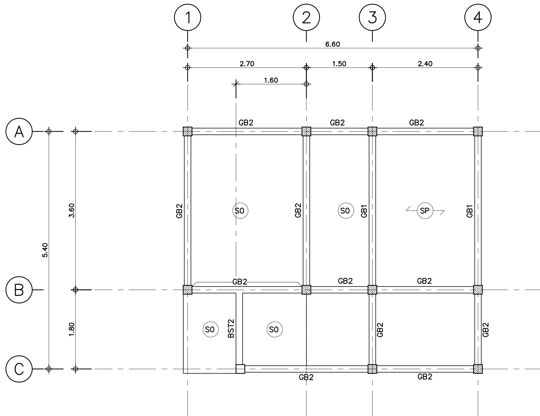
แปลน เสา, คาน, พื้นชั้น 1 มาตราส่วน 1:50
