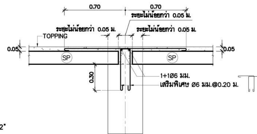
ลักษณะการวางพื้น SP ภายใน มาตราส่วน 1:20
