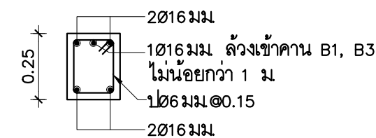
BX - BX
