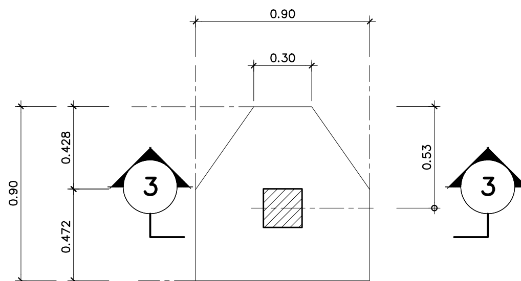
F(0.90x0.90x0.30) มาตราส่วน 1 : 20
