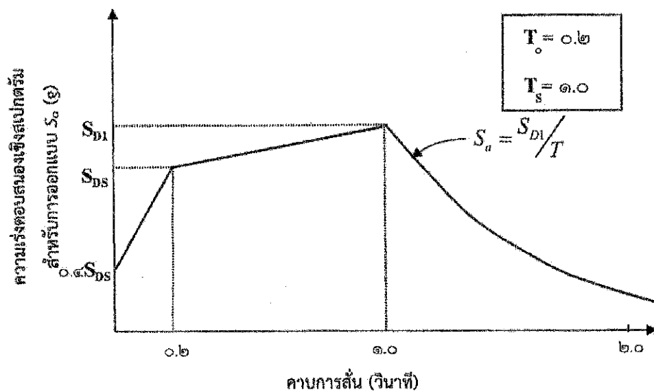
รูปที่ ก-๔ ความแรงตอบสนองเชิงสเปกตรัมสำหรับการคำนวณแรงแผ่นดินไหวด้วยวิธีเชิงพลศาสตร์ สำหรับพื้นที่นอกแอ่งกรุงเทพ ที่มีค่า S_{DI} > S_{DS}
