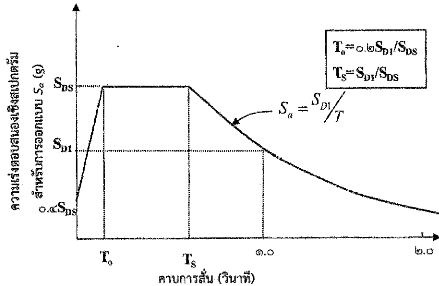
รูปที่ ก-๓ ความแรงตอบสนองเชิงสเปกตรัมสำหรับการคำนวณแรงแผ่นดินไหวด้วยวิธีเชิงพลศาสตร์ สำหรับพื้นที่นอกแอ่งกรุงเทพ ที่มีค่า S_{DI} \leq S_{DS}
