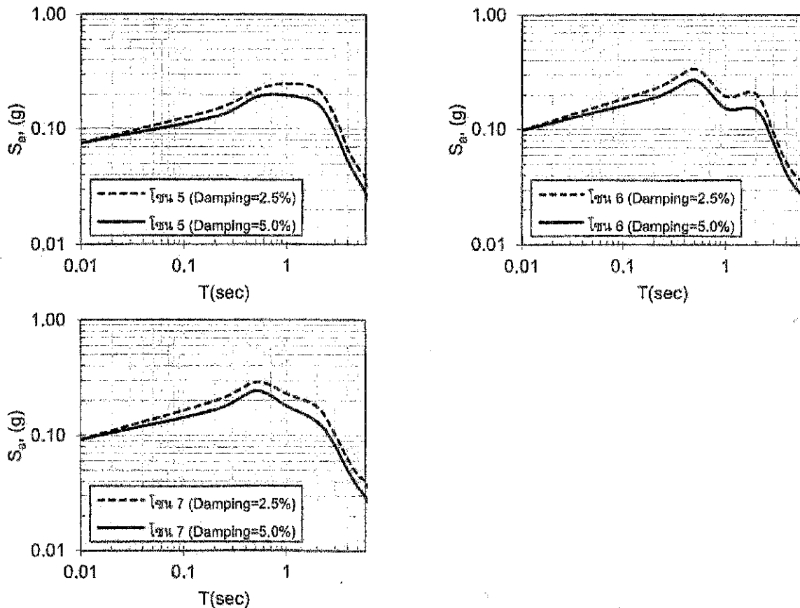
รูปที่ ก-๗ ความเร่งตอบสนองเชิงสเปกตรัมสำหรับการคำนวณแรงแผ่นดินไหวด้วยวิธีเชิงพลศาสตร์ สำหรับโซน ๑-๗ ของพื้นที่ในแอ่งกรุงเทพ
